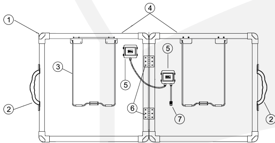
Obrázek č.1 – Technický popis solárního panelu VIKING LVP80, LVP120
